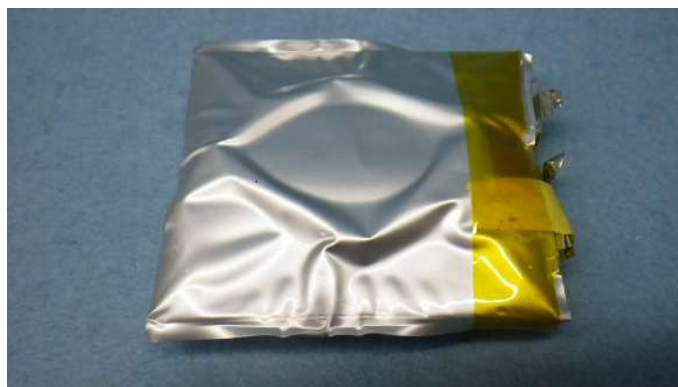
発熱し、膨れたリチウムイオンバッテリー
